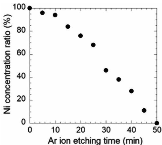
図1 11個のターゲットを利用して作製した傾斜機能性薄膜の深さ方向分析結果
