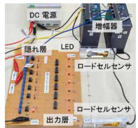
梁の上に置かれた物の重心位置の検出装置
